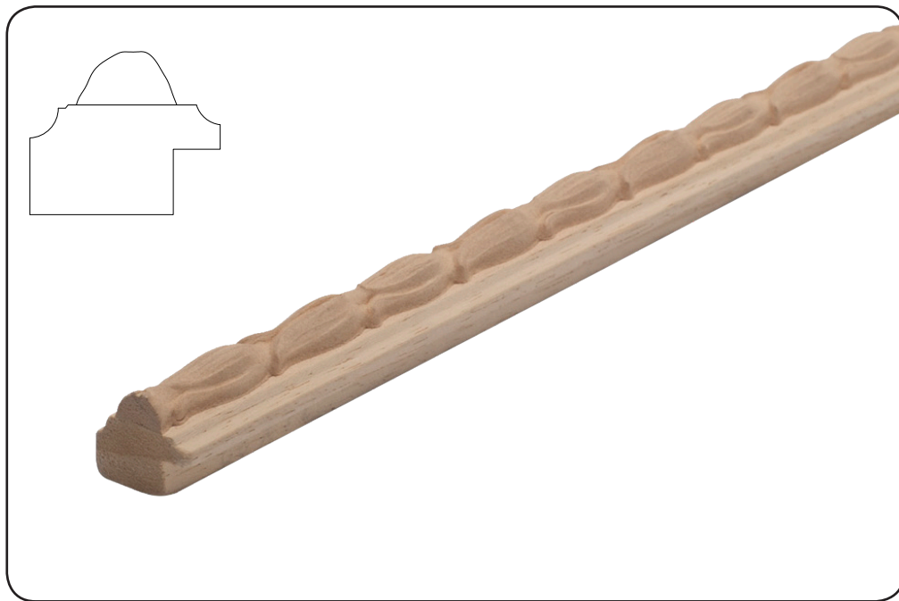
145p H 21 mm L 24 mm h Battente 9 mm
