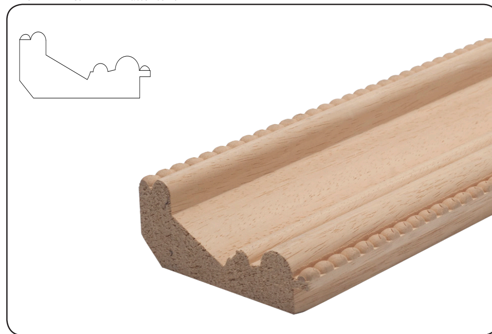
295p H 41 mm L 95 mm h Battente 12 mm
