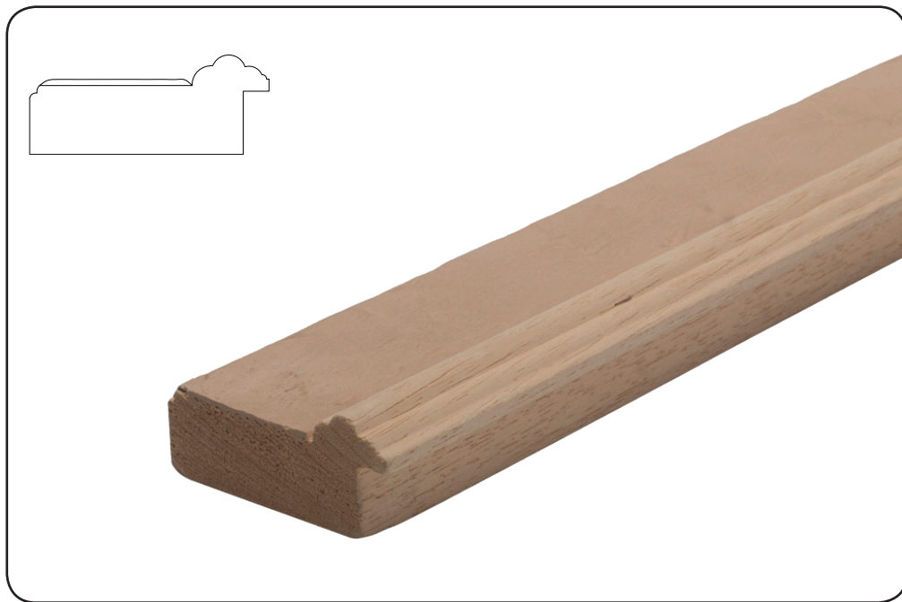
128p H 28 mm L 63 mm h Battente 18 mm
