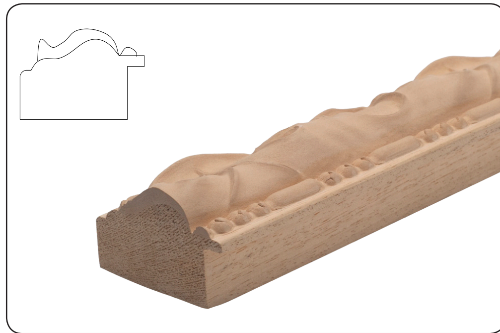
34p H 49 mm L 75 mm h Battente 27 mm
