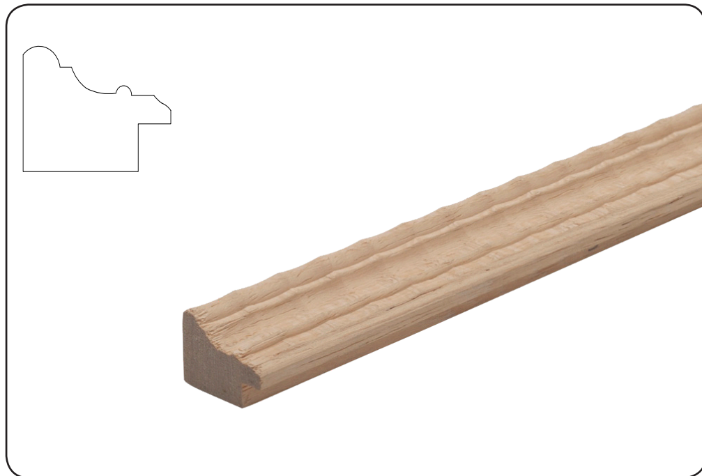
302 H 21 mm L 28 mm h Battente 9 mm
