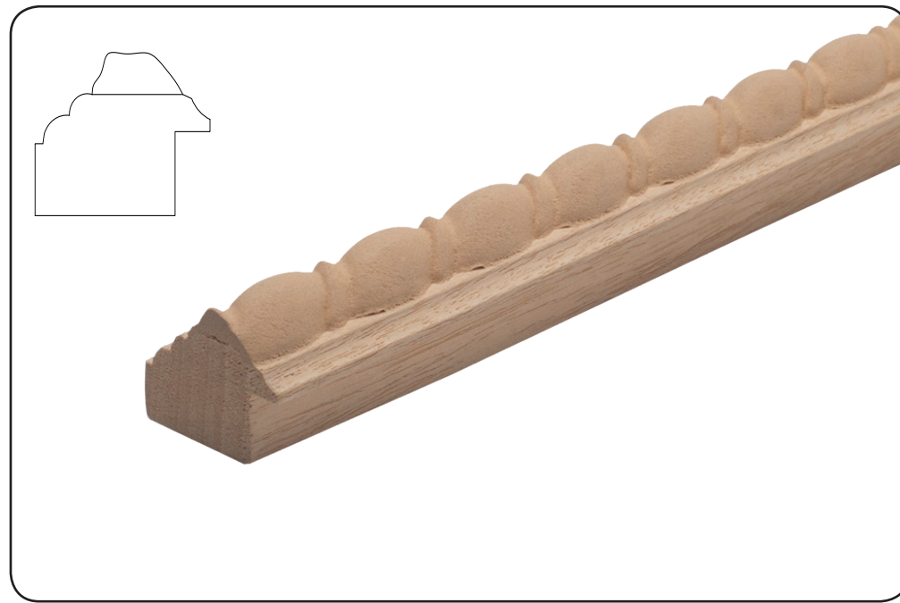
56p H 34 mm L 40 mm h Battente 17 mm
