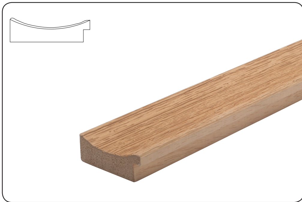
166p H 24 mm L 68 mm h Battente 15 mm
