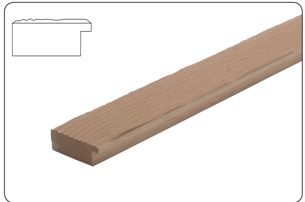
411p H 17 mm L 45 mm h Battente 10 mm
